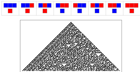
ルール30 (クラス3)
