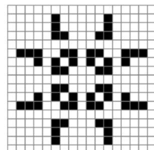
パルサーは周期3の振動子
