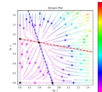
ベクトル場
