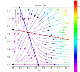
ベクトル場
