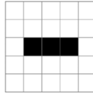
ブリンカー blinker
