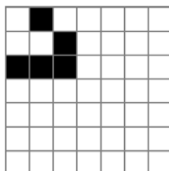
グライダー glider
