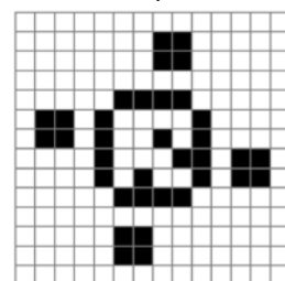
回転花火 pinwheel
