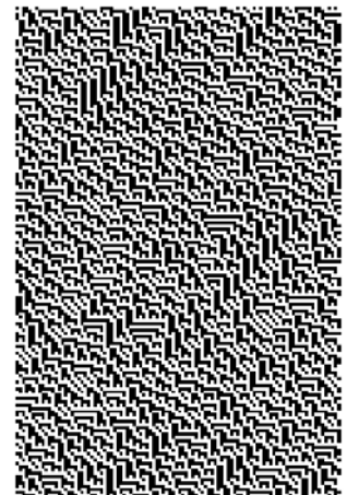
カオス
