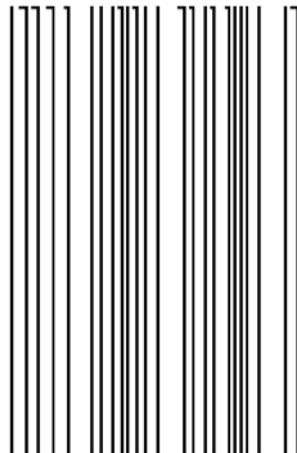
リミットサイクル
