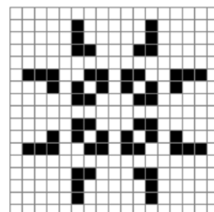
パルサーは周期3の振動子
