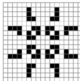
パルサーは周期3の振動子
