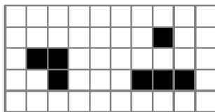
130世代後に消失
